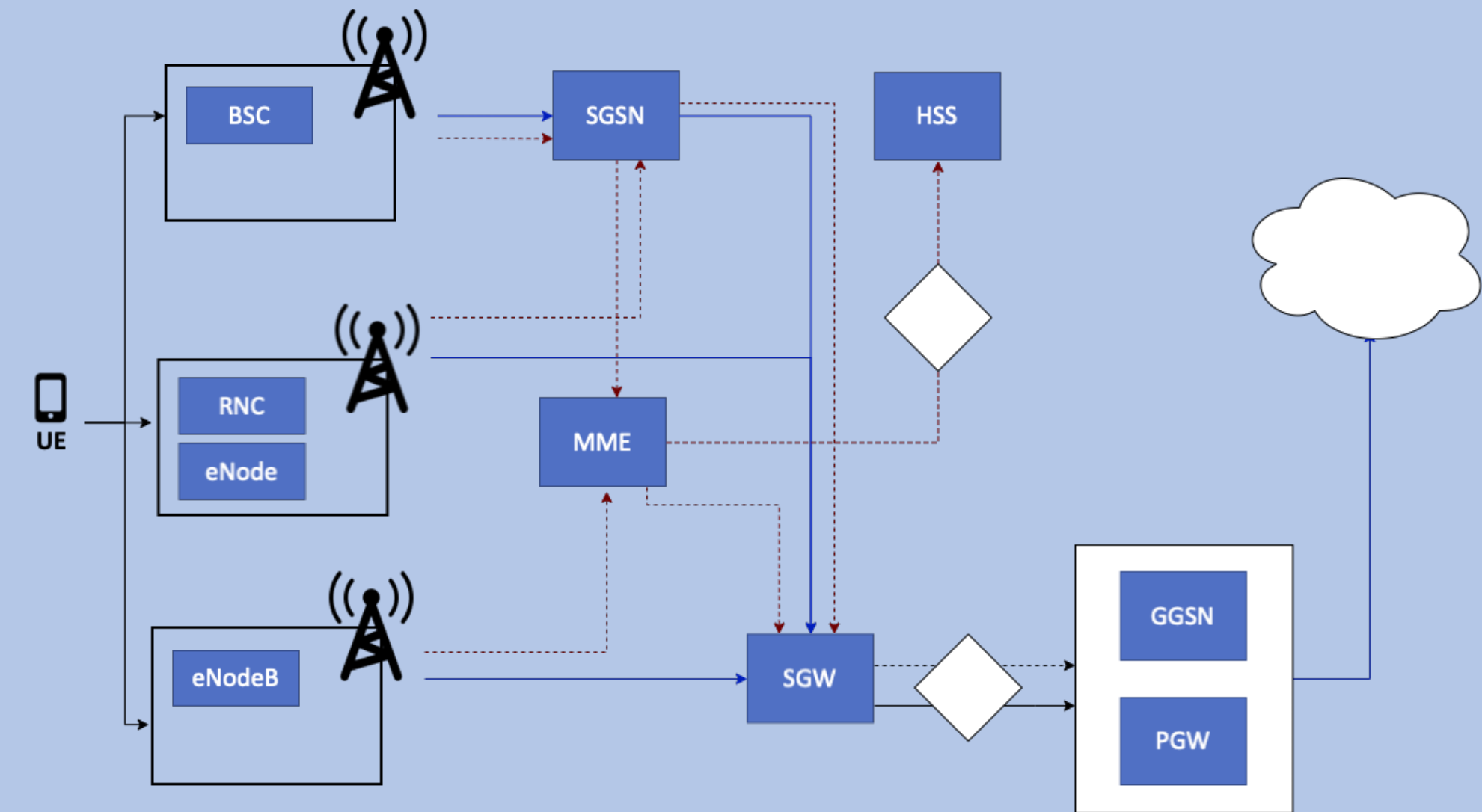
SIA 1NCE tīkla arhitektūras shēma
